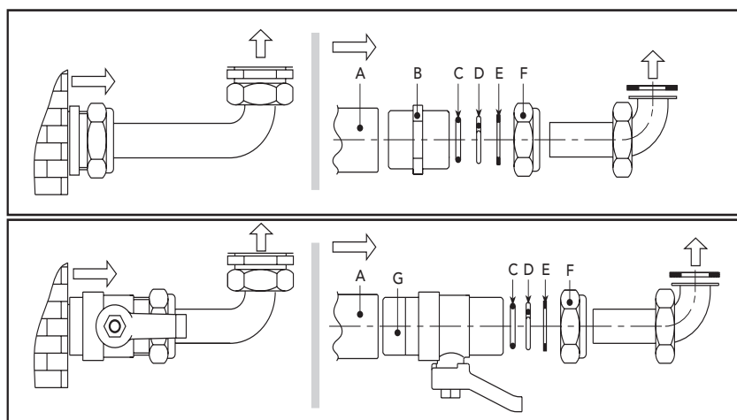
рис. 17 - Соединительный комплект
