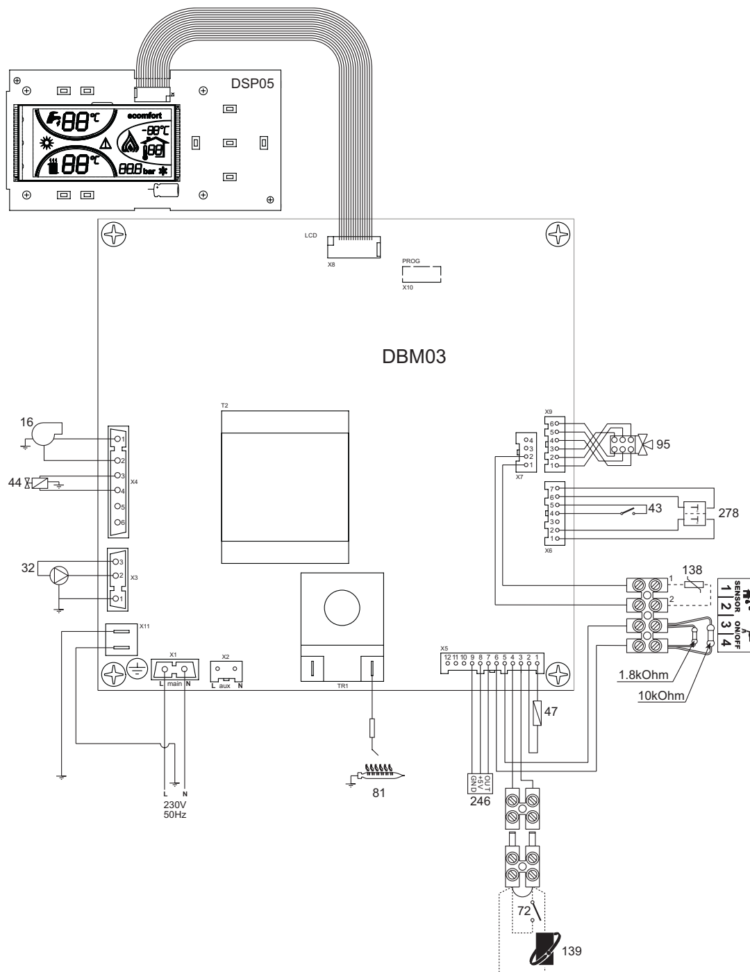
рис. 33 - Электрическая схема
