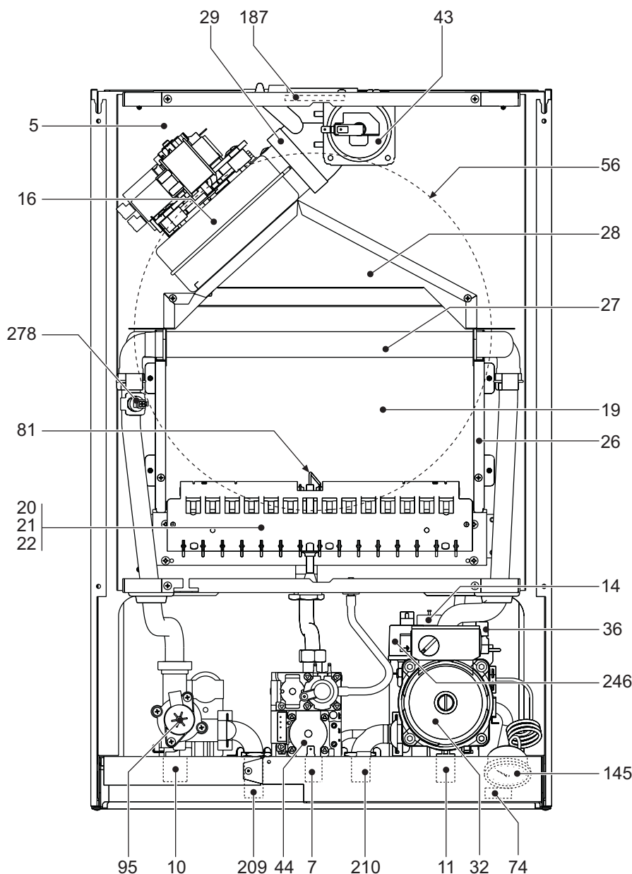
рис. 31 - Общий вид
