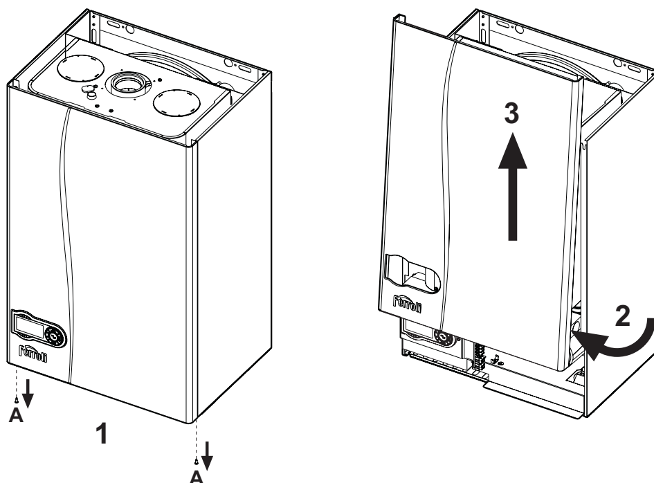
рис. 28 - Снятие кожуха
