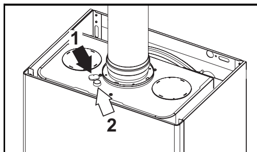
рис. 29 - Анализ продуктов сгорания
