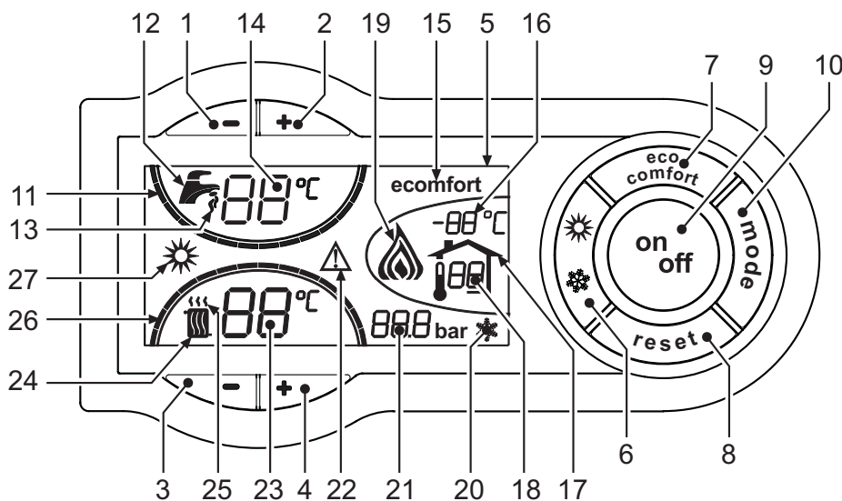
рис. 1 - Панель управления
