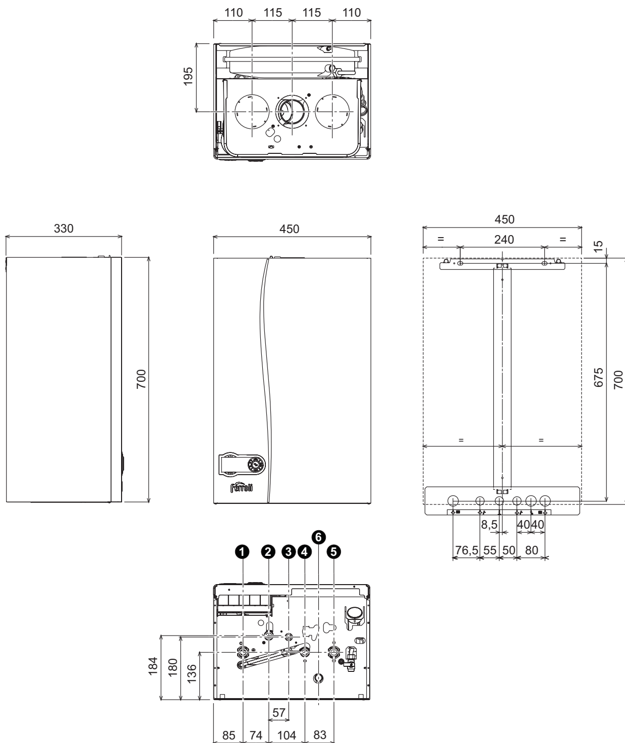
рис. 30 - Габаритные размеры и присоединения
